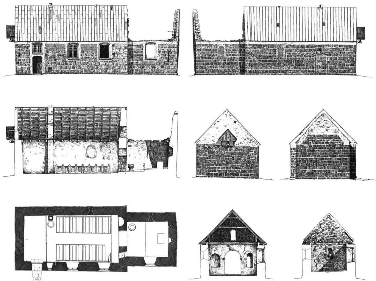
Fig. 7a-f. Opmåling afkirken efter branden 1908 ved Hother Paludan. 1:300. a. Opstalt af kirkens sydside, b. Opstalt af kirkens nordside. c. Længdesnit set mod nord. d. Opstalter af vest- og østgavl. e. Plan. f. Tværsnit gennem skib og kor set mod øst. — Vermessung von der Kirche nach dem Feuer 1908. a. Aufriß von Südwand.. b. Aufriß von Nordwand. c. Längsschnitt nach Norden. d. Aufrisse von West- und Ostgiebel. e. Grundriß. f. Querschnitt durch Schiff und Chor gegen Osten.
