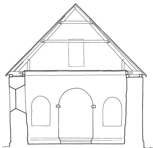
Fig. 5. Tværsnit 1:150 gennem skibet set mod øst. Målt af Peter Duun Andersen 1999 og tegnet af MN 2000.— Querschnitt durch Schiff gegen Osten.
